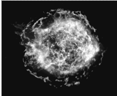
Cas A SNR X-ray Chandra
